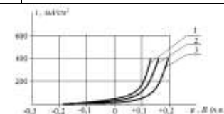
Рис. 1. Анодные потенциодинамические поляризационные кривые
